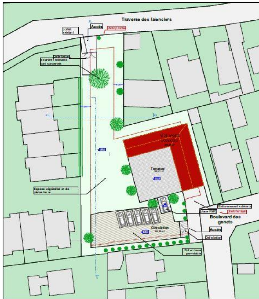
Plan Masse - Existant
